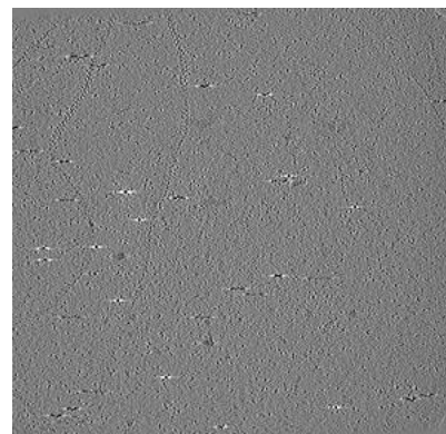
Z Index: 39
