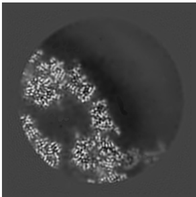
Y Index: 55
