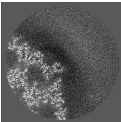
Y Index: 79
