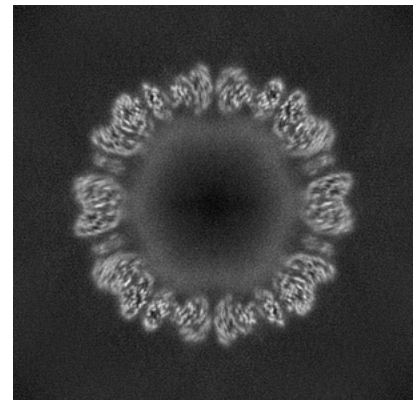
Z Index: 275
