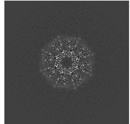
Z Index: 205
