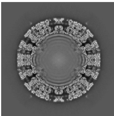
Y Index: 375
