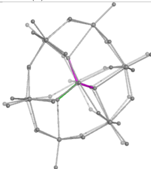
Bond angles
