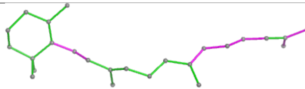
Bond angles
